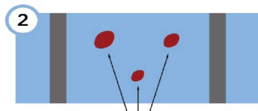
Rellene completamente la abolladura o el daño con masilla de barrera contra fuego Fire Barrier Sealant CP 25WB+ de 3M
